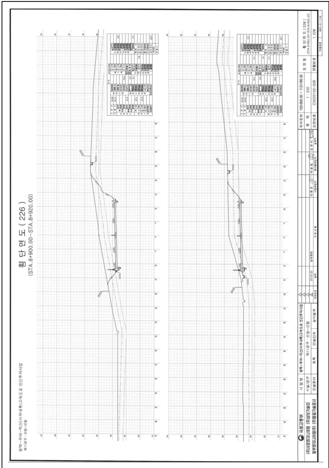
【그림 4.31.4】 횡단면도1
